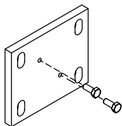
Płyta mocująca do kon- soli ściennej / uchwyty uniwersalne
