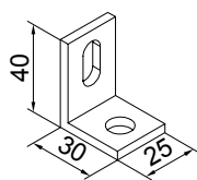
Kątownik dystansowy
