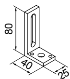
Kątownik dystansowy
