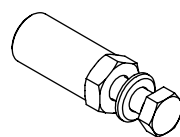
Redukcja M 10 → M 6 / SW 13
