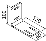
Dodatkowy kątownik do montażu niszowego
