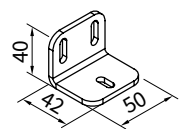
Kątownik do montażu niszowego do przewodnicy linkowej
