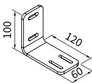
Dodatkowy kątownik do montażu niszowego
