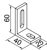
Kątownik dystansowy
