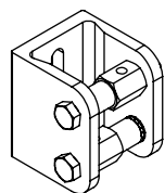
Osprzęt do podwójnego uchwyty linki
