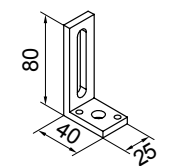
Kątownik dystansowy
