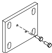
Płyta mocująca do kon- soli ściennej / uchwyty uniwersalne
