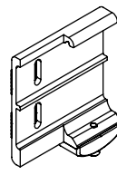
Konsola ścienna z nakładką do bocznego mocowania, lewa
