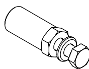
Redukcja M 10 → M 6 / SW 13
