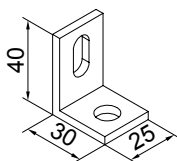
Kątownik dystansowy
